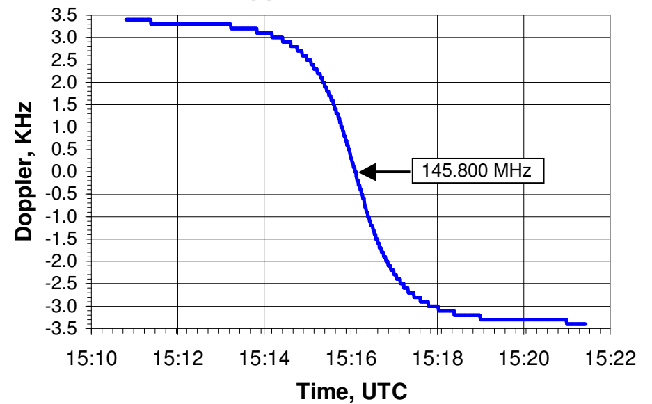
Doppler shift vs. Time
